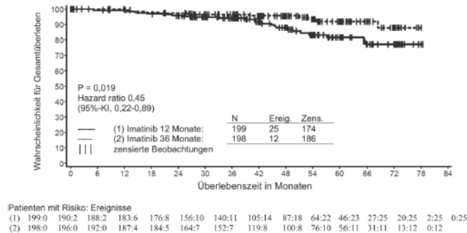
Abbildung 2 Kaplan-Meier-Schätzung für das Gesamtüberleben (ITT-Population)
