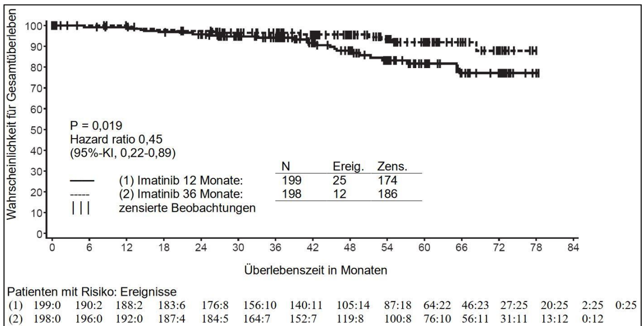
Abbildung 2: Kaplan-Meier-Schätzung für das Gesamtüberleben (ITT-Population)
