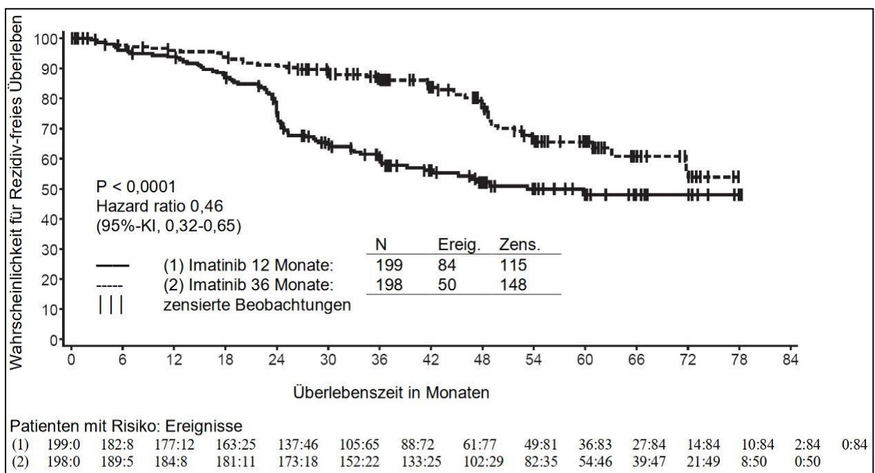
Abbildung 1: Kaplan-Meier-Schätzung für den primären Endpunkt Rezidiv-freies Überleben (ITT-Population)
