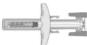
Sicherheitsspritze: Nach der Anwendung (mit aktiviertem Kanülenschutzmechanismus)
