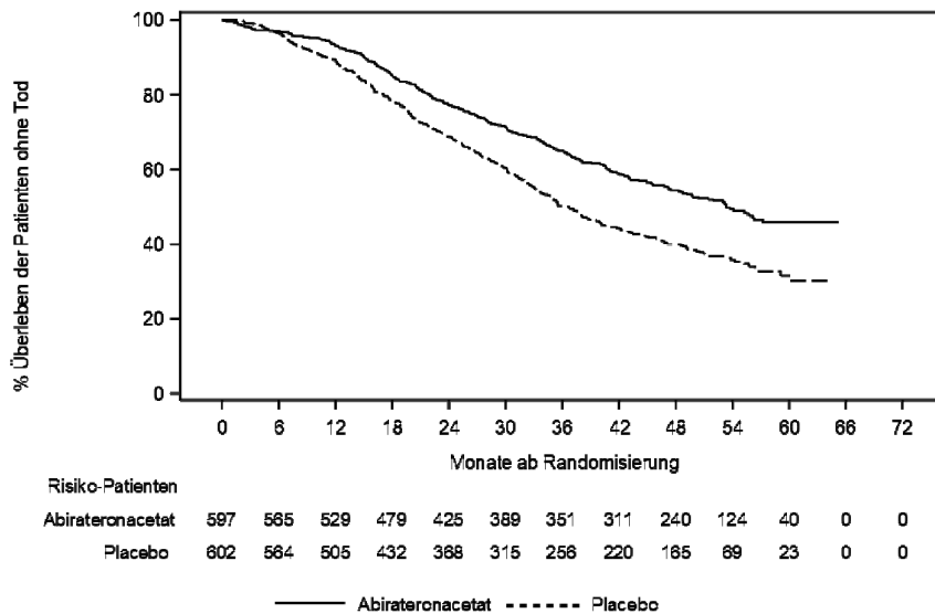
Abbildung 2: Kaplan-Meier-Kurve des Gesamtüberlebens; Intent-To-Treat-Population in Studie PCR3011
