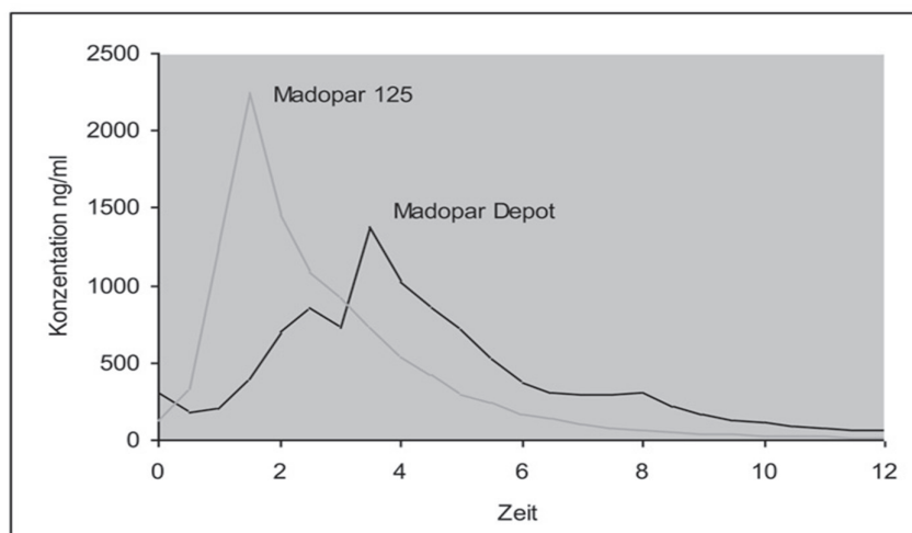
Abb. 1: Mittlere Plasmaspiegelverläufe von Madopar 125 mg, Hartkapseln, und Madopar Depot, Hartkapseln retardiert, in einem Konzentrations-Zeit-Diagramm.
