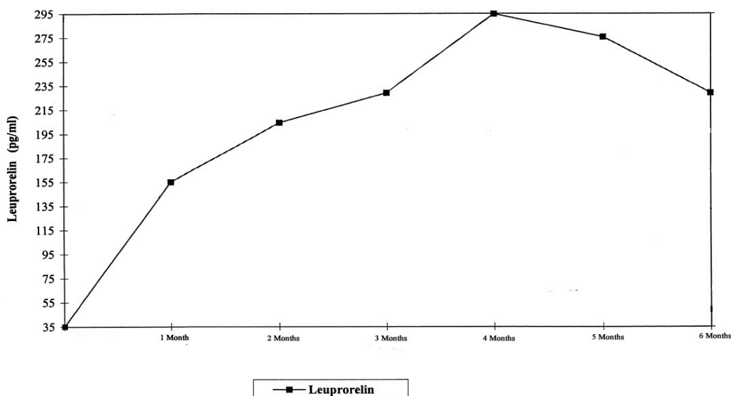
Abb.4: Leuporelinspiegel im Serum während der ersten 6 Monate nach Applikation von Klebrocid 3-Monats-Depot bei Kindern und Jugendlichen mit CPP (2 s.c. Injektionen, n = 42-43).
